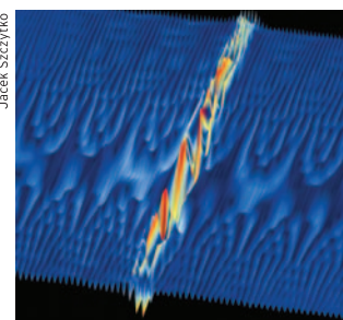
De la lumière en interaction avec un trou de la taille d'un atome dans un cristal
